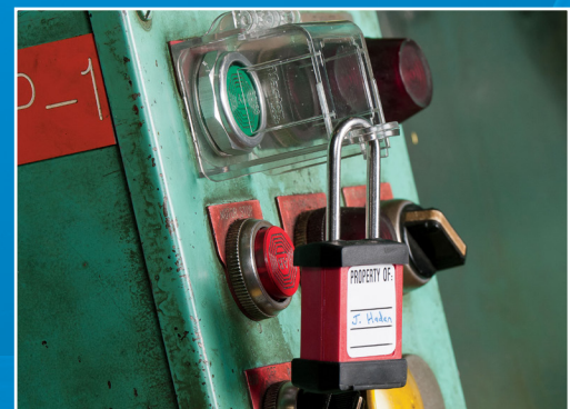
S2153 montiert mit S31REDCOV.
